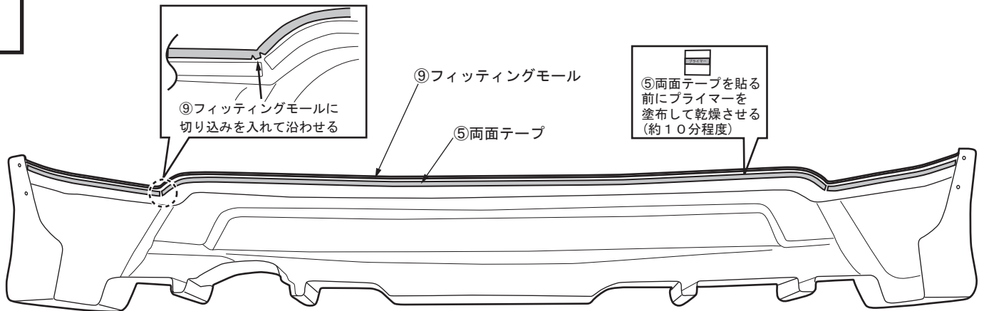
①リアハーフスポイラー裏面
